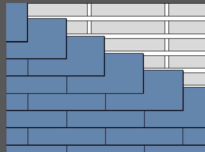
Halfsteensverband (dak en gevel) Dekking zoals toegepast voor dit project
