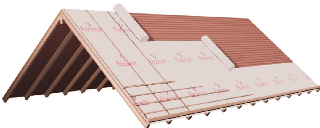
Fig. 2: DUO LONGLIFE EXTRA geplaatst op houten bebording
