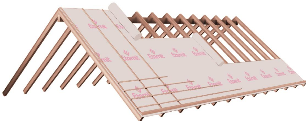
Fig. 1: DUO LONGLIFE EXTRA geplaatst op de kepers
