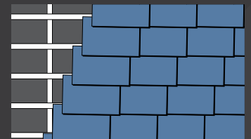
Enkelvoudige horizontale dekking (dak en gevel)
