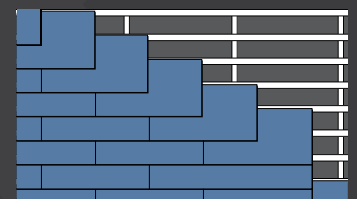
Halfsteensverband (dak en gevel)
