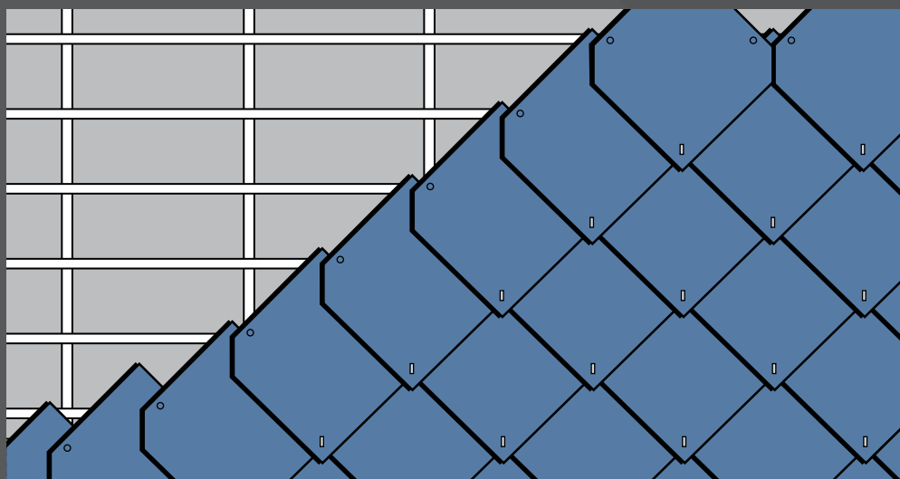
Ruitleien - Klassieke plaatsing (dak en gevel) Dekking zoals toegepast voor dit project
